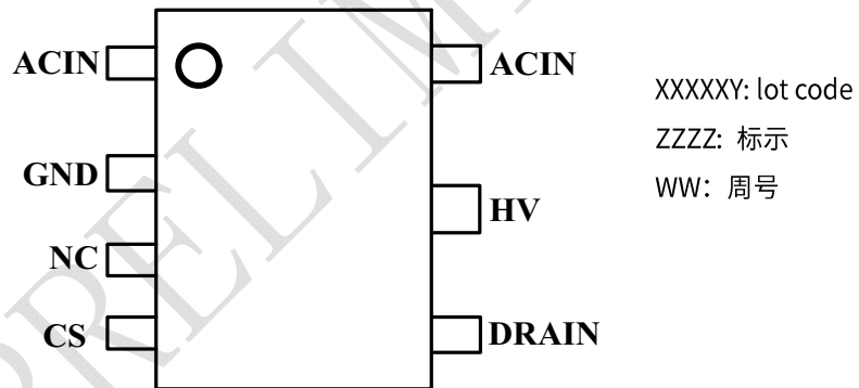
图 7 管脚封装图
