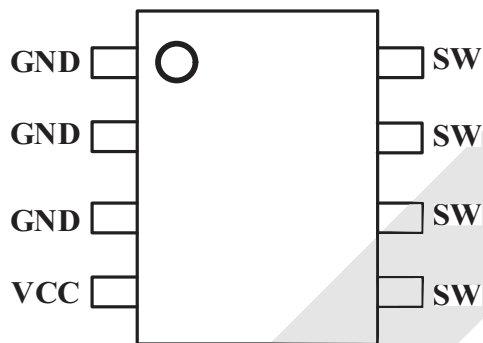
图 2 封装
